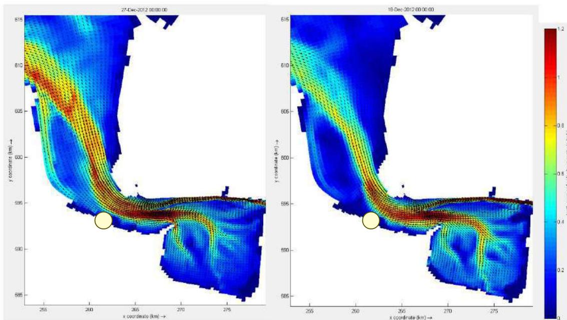
Figuur 3.2 Benadering van de maximale stroomsnelheden tijdens eb (links) en tijdens vloed (rechts) op basis van het Eems-Dollard model. Bron: Cumulatieve effecten baggeren en verspreiden op habitattype H1130 in het Eems estuarium. Deel 1: Abiotische effecten , Deltares 2022
